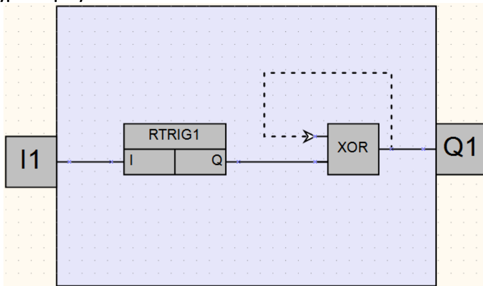
Малюнок 2 – Структурна (функціональна) схема макросу
