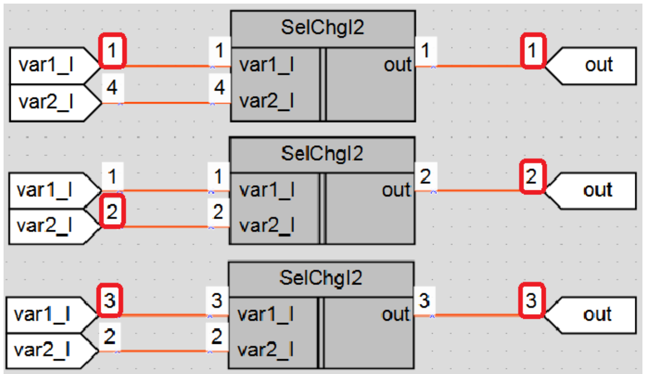
Малюнок 2 – Приклад роботи макросу
